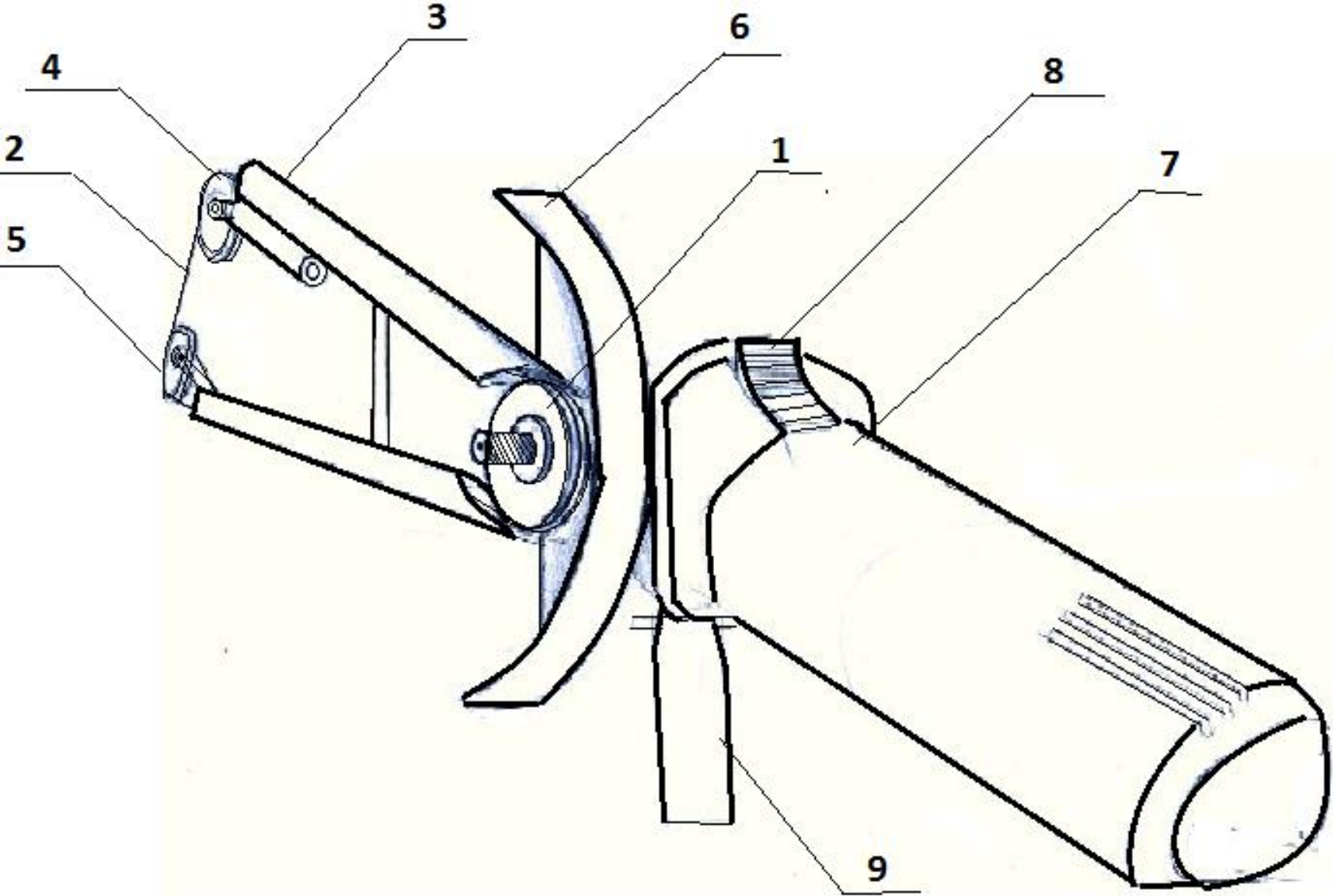
АЛМАЗНО КАНАТНЫЙ УСТРОЙСТВО АКУ-1
